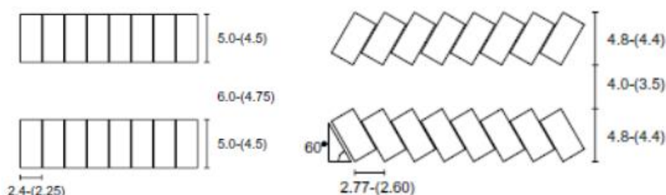
Figura 40. Dimensiones recomendadas y mínimas de plazas de estacionamiento en batería. Fuente: Elaboración propia.
