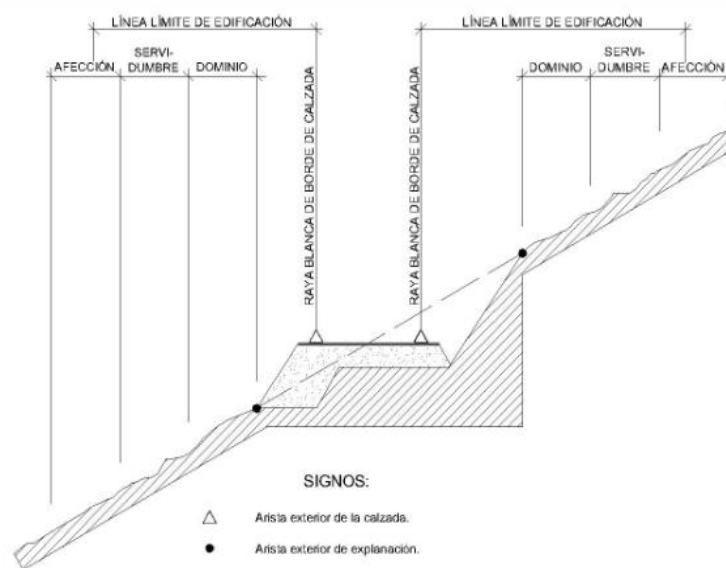
Figura 12. Franjas de protección y línea límite de la edificación. Fuente: Elaboración propia a partir de la Ley de Carreteras de Canarias.
