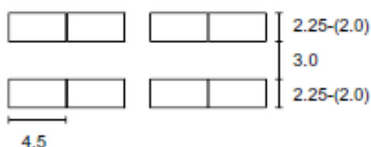
Figura 39. Dimensiones recomendadas y mínimas de plazas de estacionamiento en línea.
